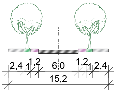
Слика 6 Пресек на сервисна улица „Димитар Влахов“
