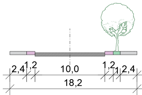
Слика 7 Пресек на сервисна улица „Партизанска“
