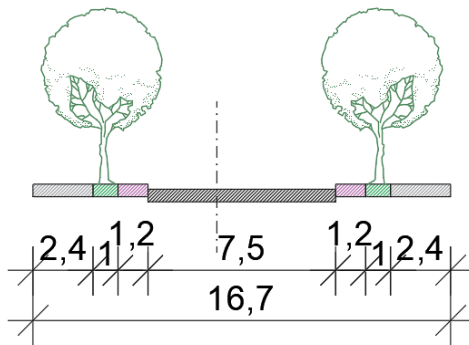
Слика 8 Пресек на станбена улица „Ванчо Николески“
