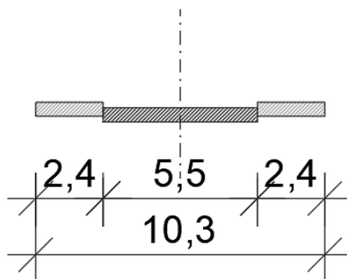
Слика 9 Пресек на станбена улица „Серафим Китаноски“
